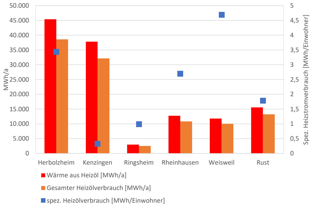
Abbildung 34: Übersicht gesamter und spezifischer Heizölverbrauchs
