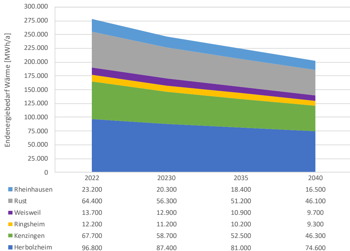
Abbildung 64: Nutzenergieverbrauchsentwicklung Konvoi
