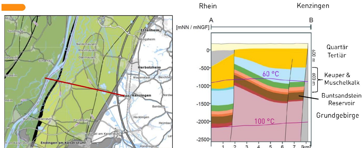
Abbildung 49: Schichtprofil Oberrheingraben, Quelle: EnBW, (GeoRG, 2013)
