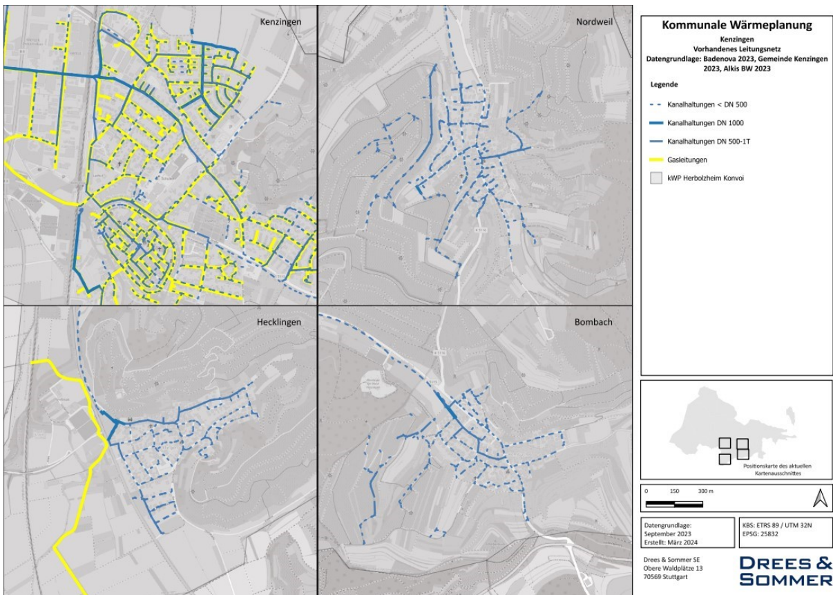
Abbildung 54: Leitungsnetze Kenzingen
